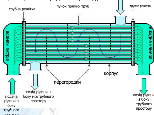
Прямотрубний теплообмінник (один прохід з боку трубного простору)
